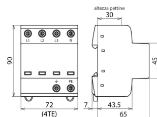
Dimensioni DSH TT 255
