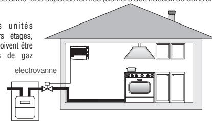
Fig. 8 Exemple d'installation
