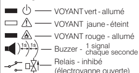
Fig. 4 - État d' "alarme présence de gaz"
