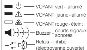
Fig. 6 - Signalisation de pannes et dysfonctionnements
