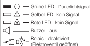
Abb. 3 - Betriebszustand "Normalbetrieb"
