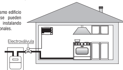
Fig. 8 Ejemplo de instalación
