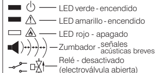
Fig. 6 - Señalización de fallos y defectos de funcionamiento
