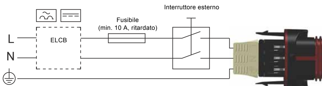
Fig. 17 Esempio di collegamento tipico, 1 x 230 V \pm 10 %, 50/60 Hz, PE
