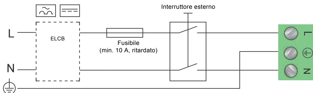
Fig. 16 Esempio di collegamento tipico, 1 x 230 V \pm 10 %, 50/60 Hz, PE
