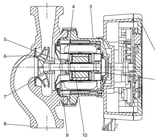
Fig. 14 Versione filettata con canotto separatore in acciaio inox
